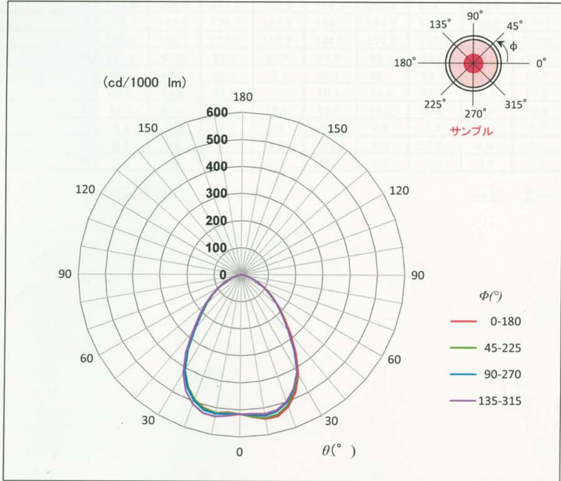
図 1 配光曲線 (cd/1000 lm)
